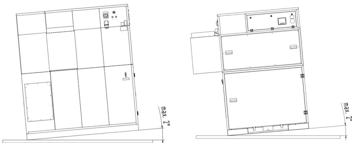
Рис. 11: Установка
